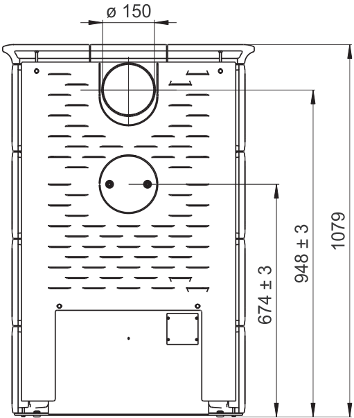
Výška osy zadního odvodu spalin (mm) - Alternativy Rauchrohrabgang hinten (mm) - Alternativen Height of the rear outlet (mm) - Alternatives
